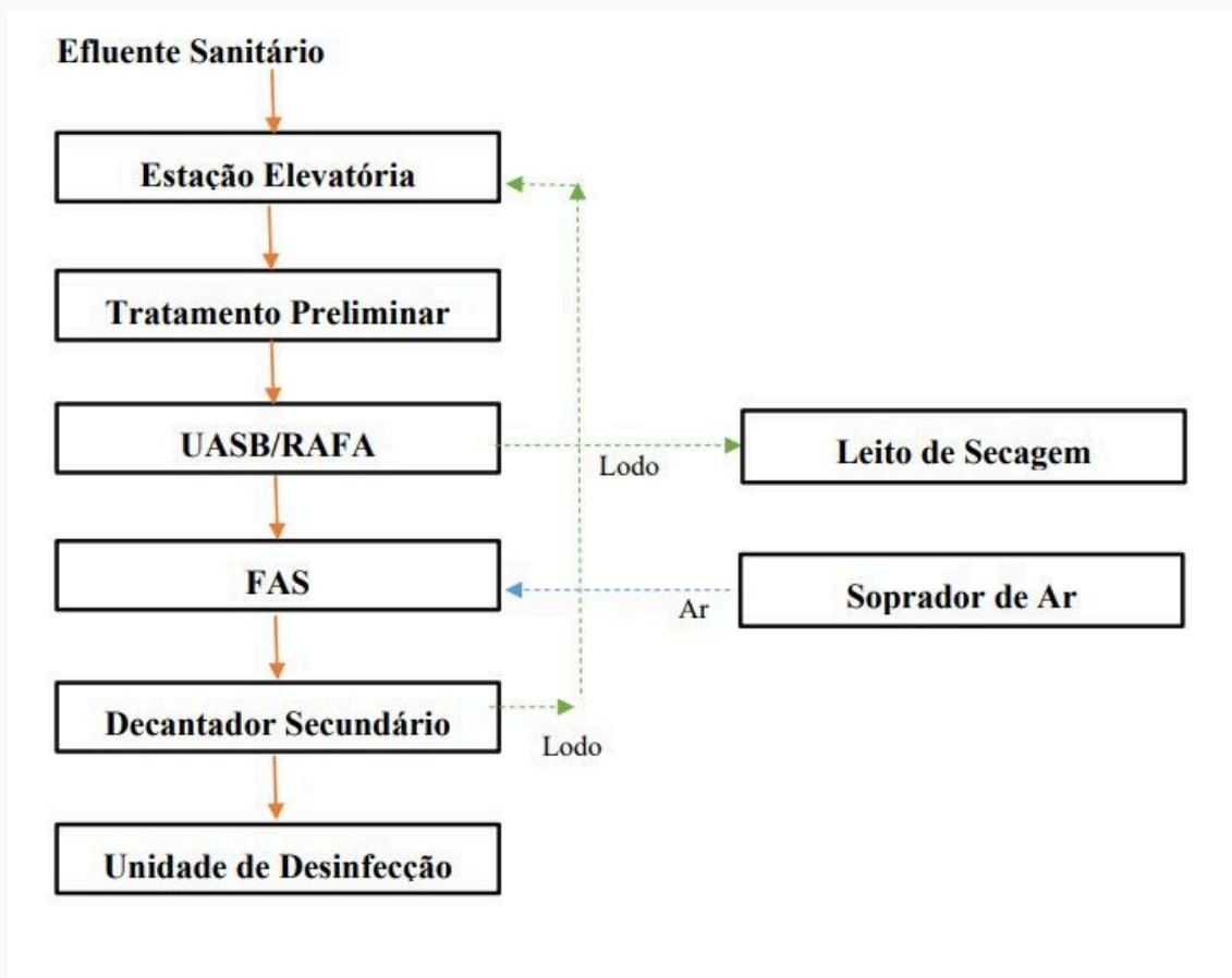
Figura 1 - Fluxograma da Estação de Tratamento de Esgoto
